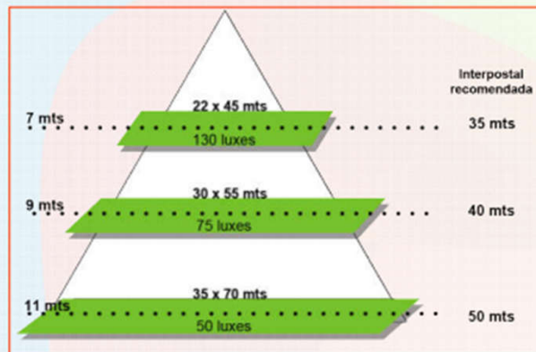
Simulación Iluminación en calle secundaria
